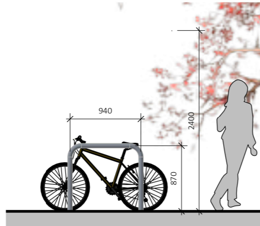
4 Cross Section A-A 1 : 50
