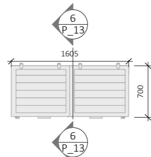
5 Bins Roof Plan 1 : 50
